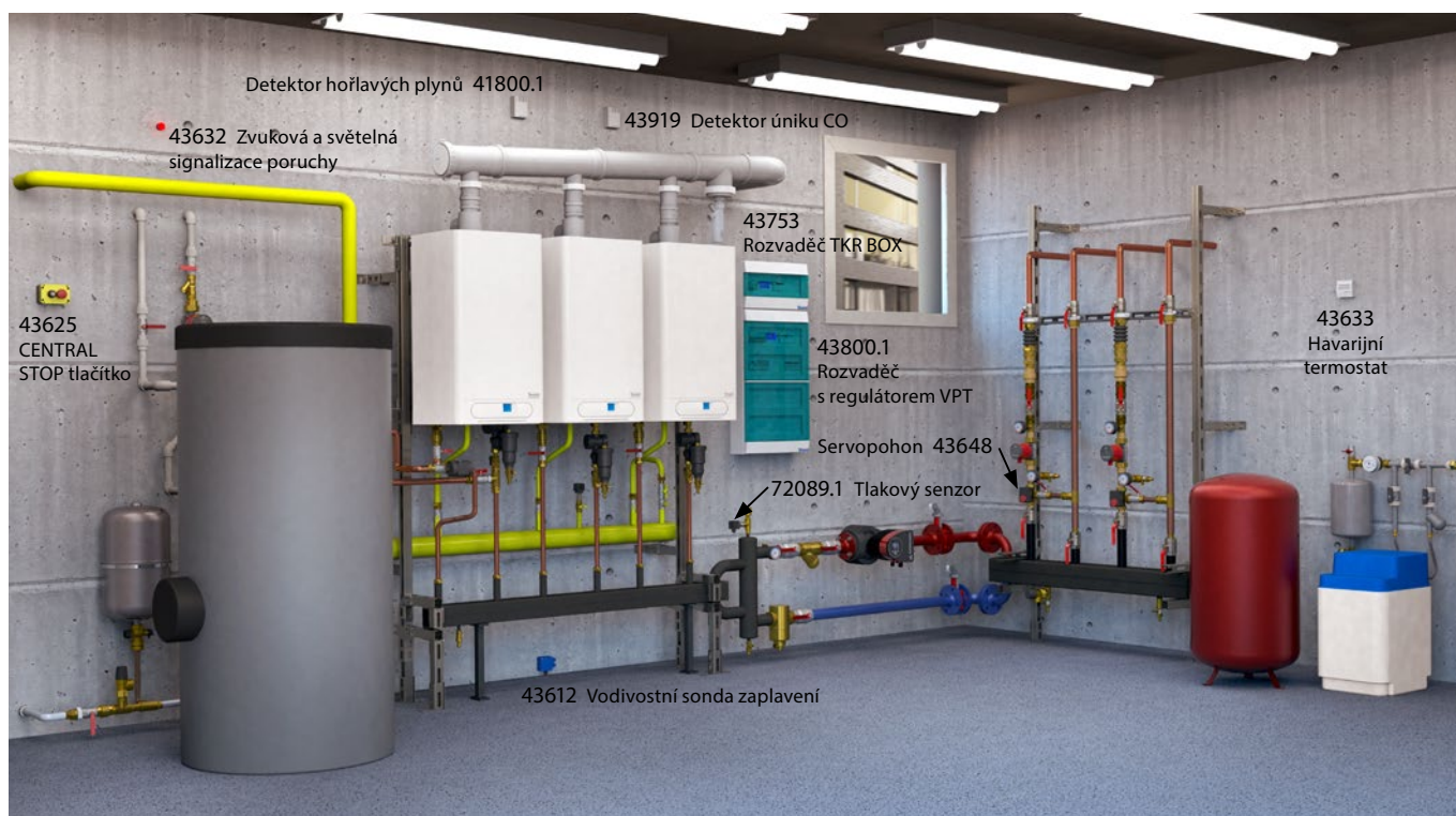
Příklad využití regulátoru THERM VPT/R v kotelně
